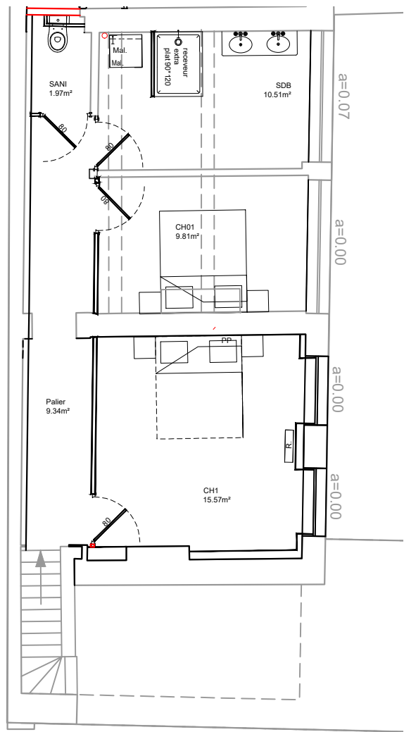
EXTRAIT PLAN REZ DE CHAUSSEE
